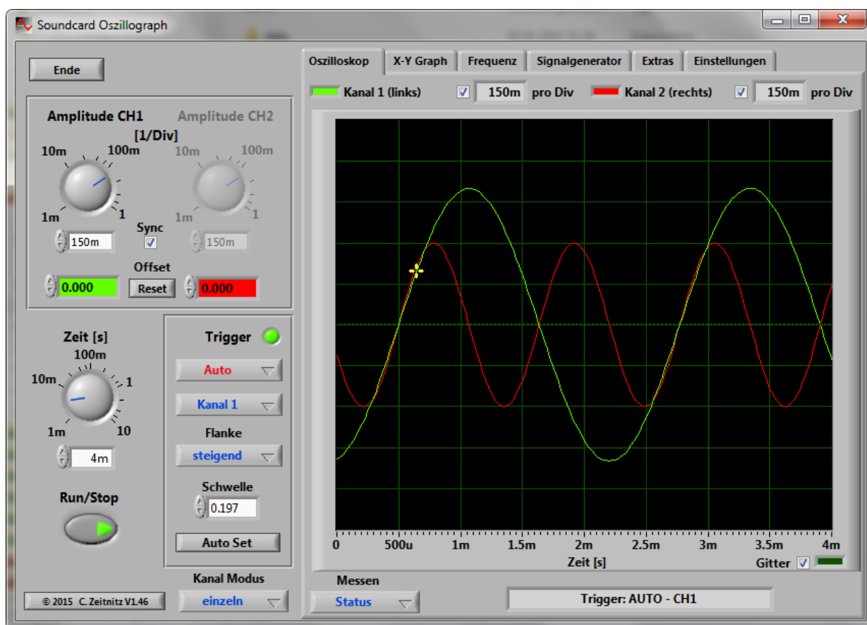
Abbildung 1: Der Soundkarten-Oszillograph
